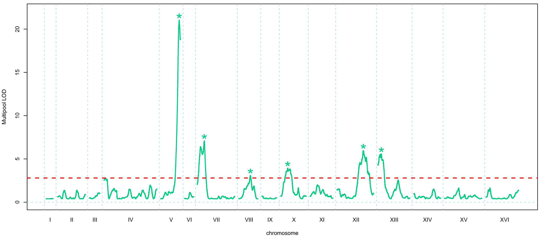
GPD1_a_0_1_4 GPD1_a_1_1_4
